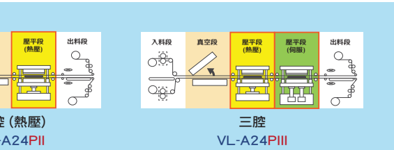
預貼機 入料段 真空段 壓平段 (熱壓) 壓平段 (伺服) 出料段
