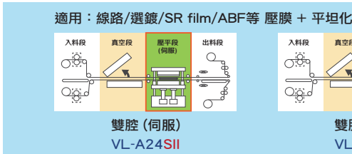
預貼機 入料段 真空段 壓平段 (熱壓) 壓平段 (伺服) 出料段
